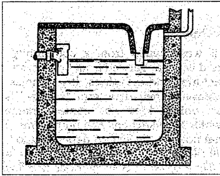
FIG. 11 Aqua privy
