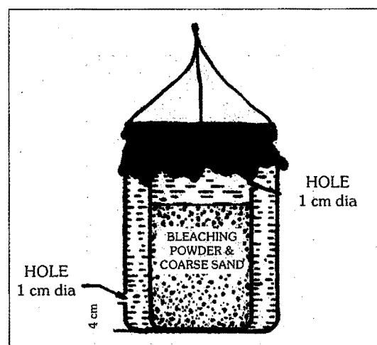
FIG. 10 Double pot
